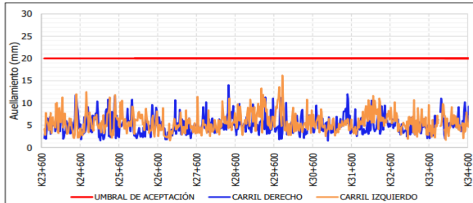
Figura 9 Evaluación E2 Ahuellamiento UF1A
