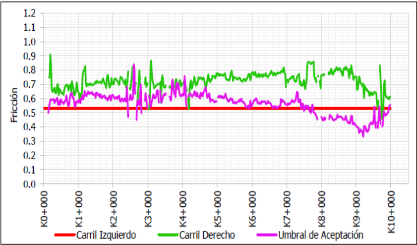
Figura 33 Comportamiento indicador E4 UF3A
