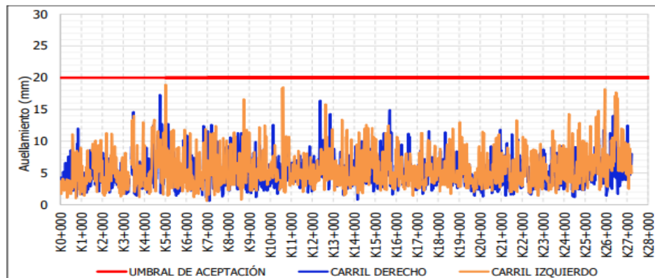
Figura 10 Evaluación E2 Ahuellamiento UF1B.
