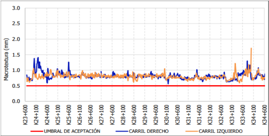
Figura 13 Evaluación E5 Textura UF1A
