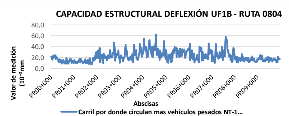
Figura 17 Evaluación E16 Capacidad Estructural UF1B
