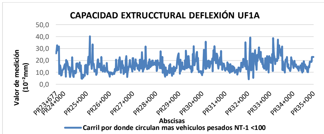
Figura 16 Evaluación E16 Capacidad Estructural UF1A
