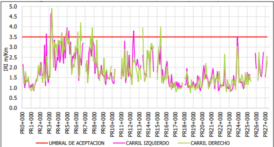
Figura 8 Evaluación E1 Iri UF1B.
