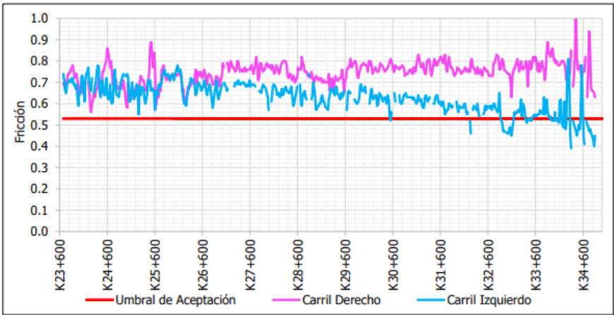
Figura 11 Evaluación E4 Fricción Transversal UF1A
