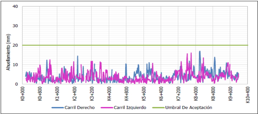
Figura 31 Evaluación E2 UF3A
