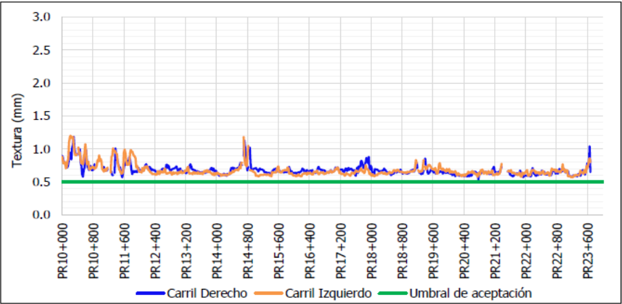
Figura 25 Evaluación E5 Textura UF2B
