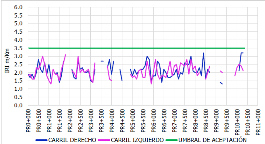
Figura 20 Evaluación E1 Iri UF2A
