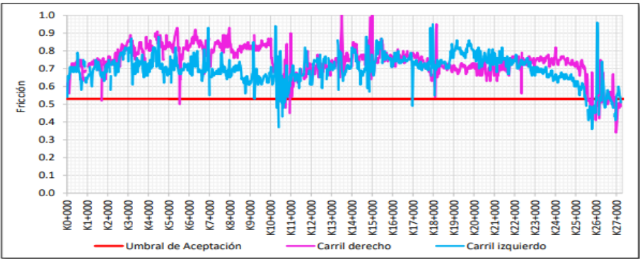
Figura 12 Evaluación E4 Fricción Transversal UF1B
