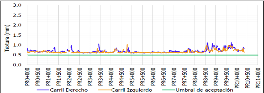
Figura 24 Evaluación E5 Textura UF2A
