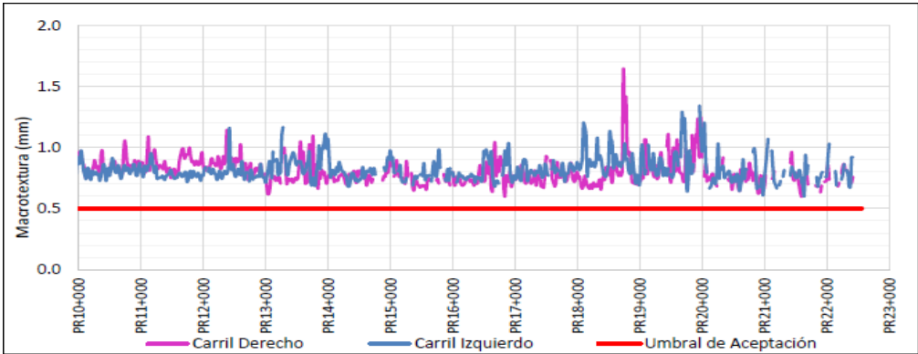
Figura 36 Comportamiento indicador E5 UF3A
