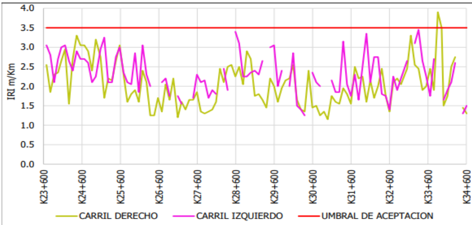
Figura 7 Evaluación E1 Iri UF1A
