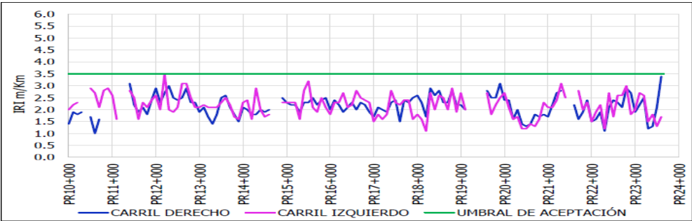
Figura 21 Evaluación E1 Iri UF2B.
