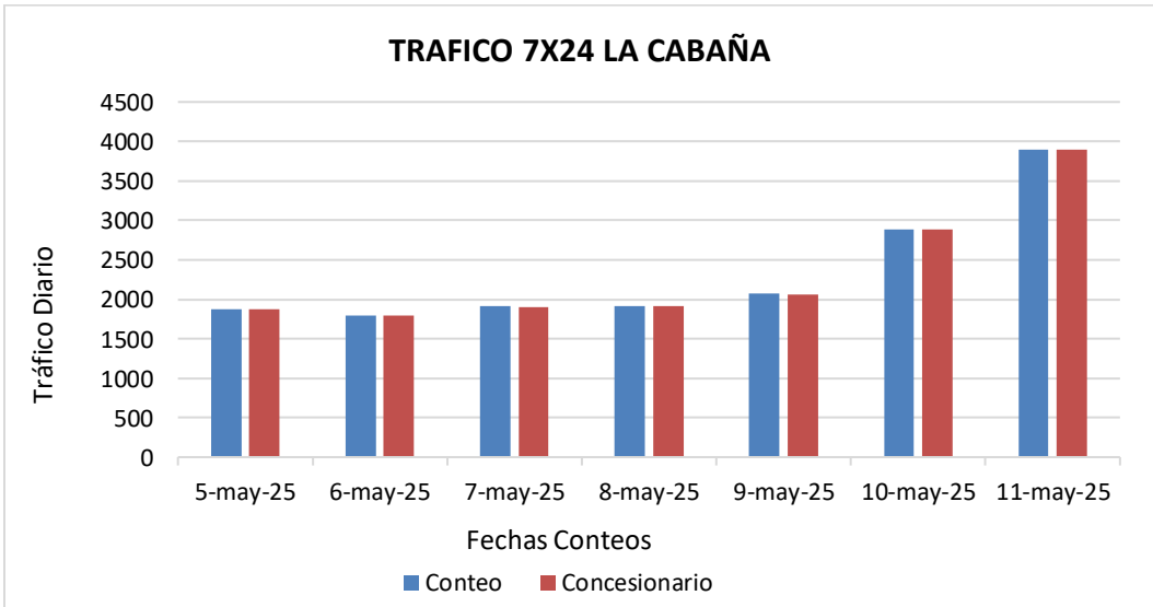
Figura 58 Comparativo Aforo 7x24 Peaje La Cabaña.
