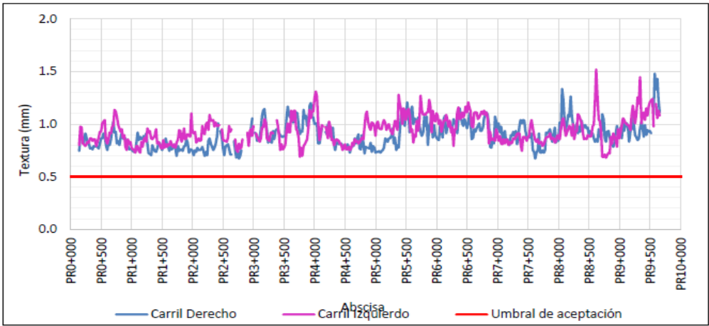
Figura 35 Comportamiento indicador E5 UF3A
