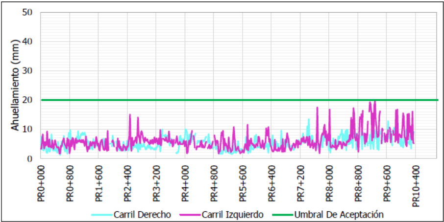
Figura 22 Evaluación E2 Ahuellamiento UF2A.
