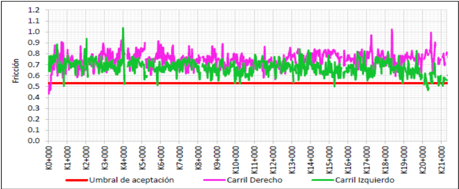
Figura 34 Comportamiento indicador E4 UF3B
