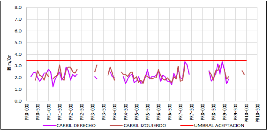
Figura 29 Evaluación E1 UF3A
