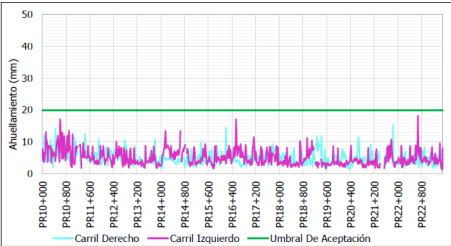
Figura 23 Evaluación E2 Ahuellamiento UF2B.
