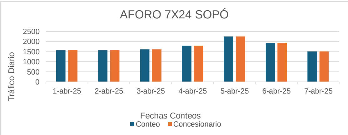
Figura 57 Comparativo Aforo 7x24 Peaje Sopó
