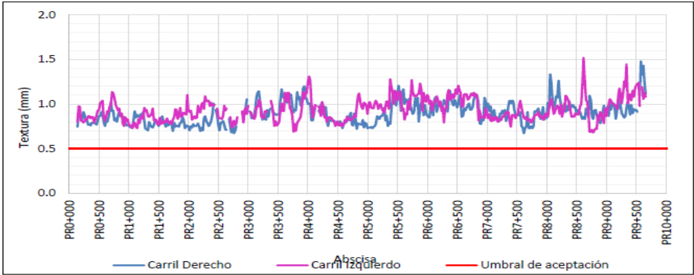
Figura 35 Comportamiento indicador E5 UF3A
