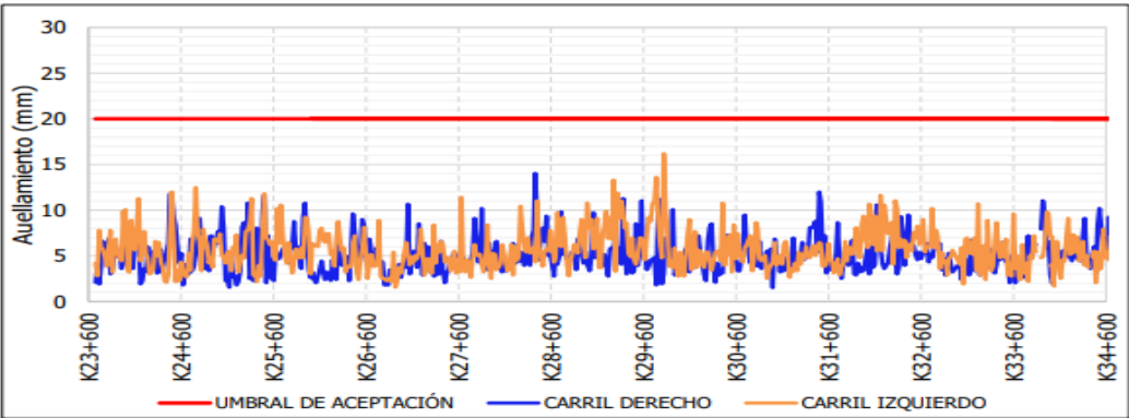
Figura 9 Evaluación E2 Ahuellamiento UF1A
