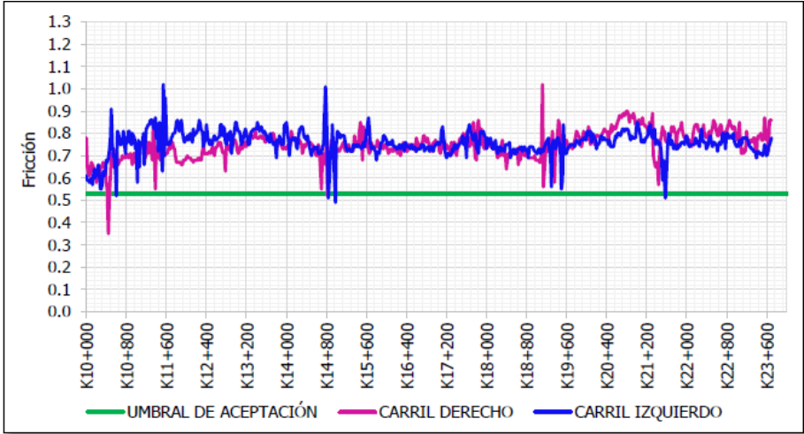
Figura 26 Evaluación E4 Fricción UF2B.
