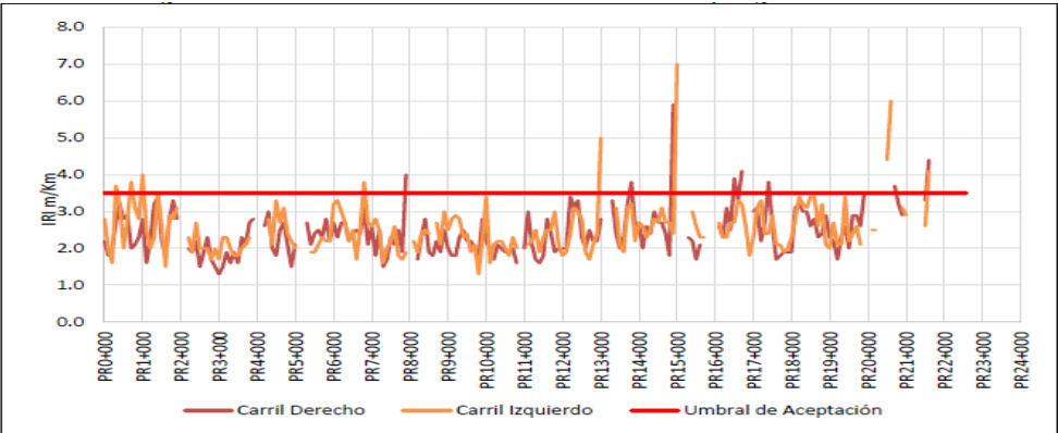
Figura 30 Evaluación E1 UF3B
