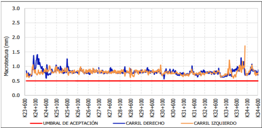
Figura 13 Evaluación E5 Textura UF1A
