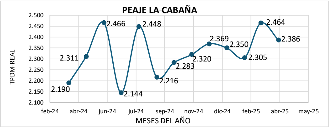
Figura 53 Tráfico promedio mes a mes peaje LA CABAÑA
