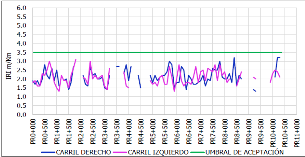
Figura 20 Evaluación E1 Iri UF2A
