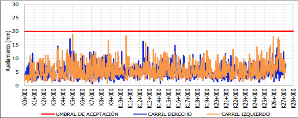
Figura 10 Evaluación E2 Ahuellamiento UF1B.
