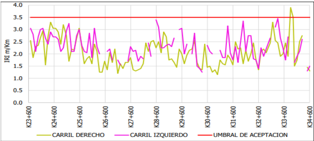
Figura 7 Evaluación E1 IRI UF1A
