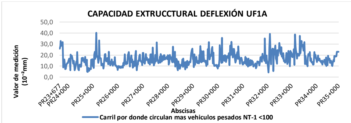
Figura 16 Evaluación E16 Capacidad Estructural UF1A
