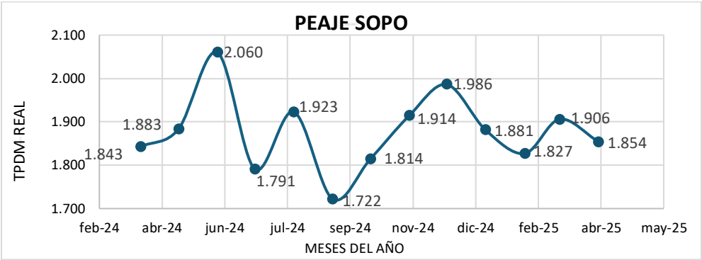
Figura 51 Tráfico promedio mes a mes peaje SOPÓ.
