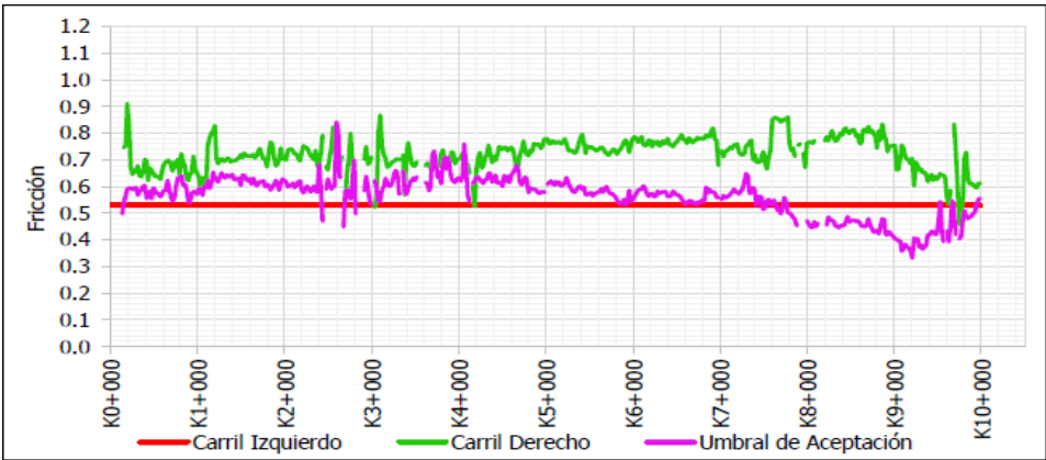
Figura 33 Comportamiento indicador E4 UF3A
