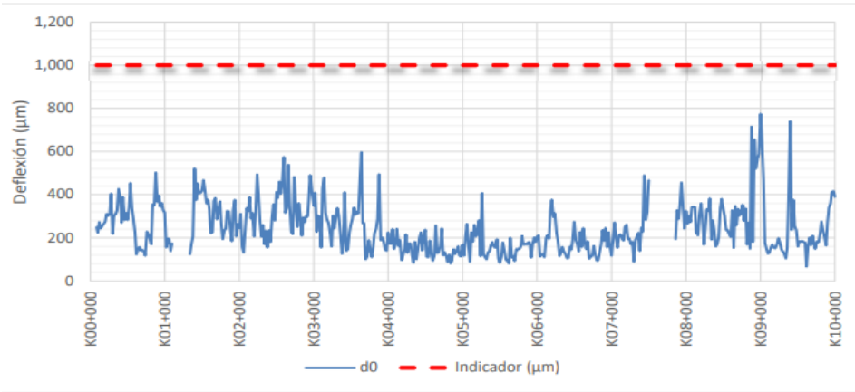
Figura 38 Evaluación E16 UF3A
