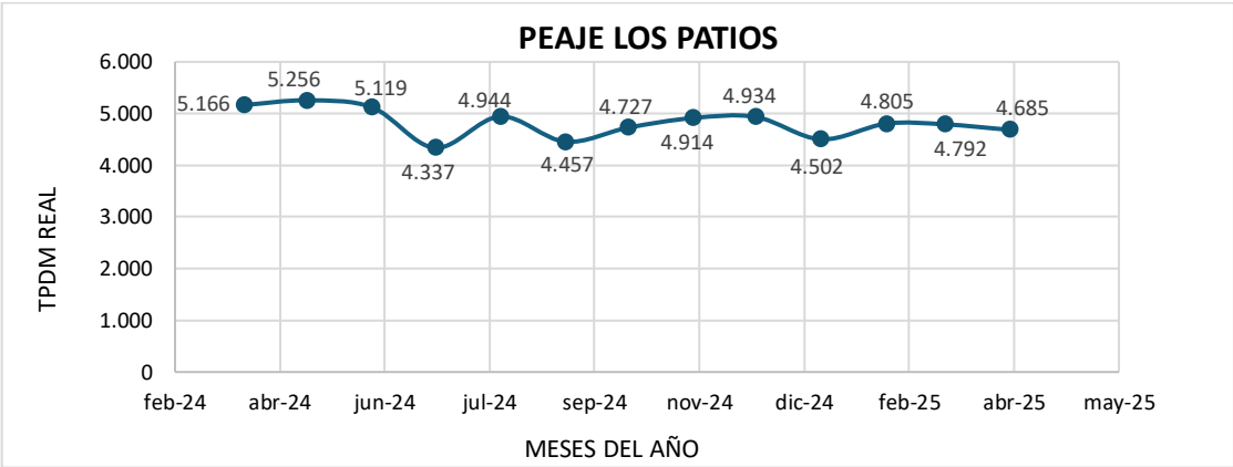
Figura 55 Tráfico Promedio Mes A Mes Peaje De Los Patios
