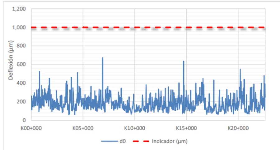
Figura 39 Evaluación E16 UF3B
