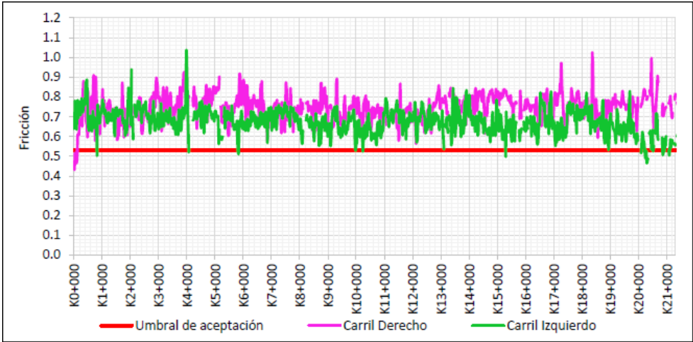
Figura 34 Comportamiento indicador E4 UF3B
