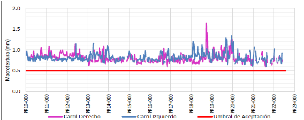
Figura 36 Comportamiento indicador E5 UF3A
