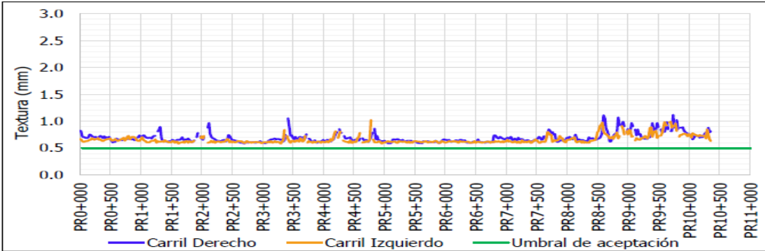
Figura 24 Evaluación E5 Textura UF2A
