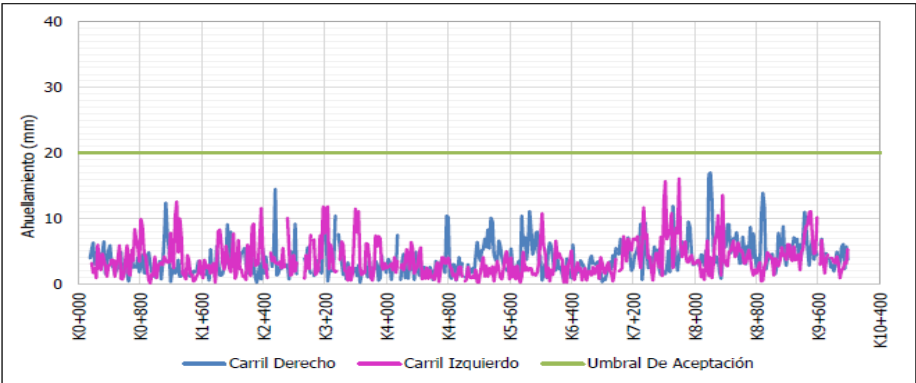
Figura 31 Evaluación E2 UF3A
