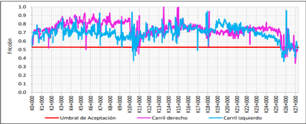
Figura 12 Evaluación E4 Fricción Transversal UF1B
