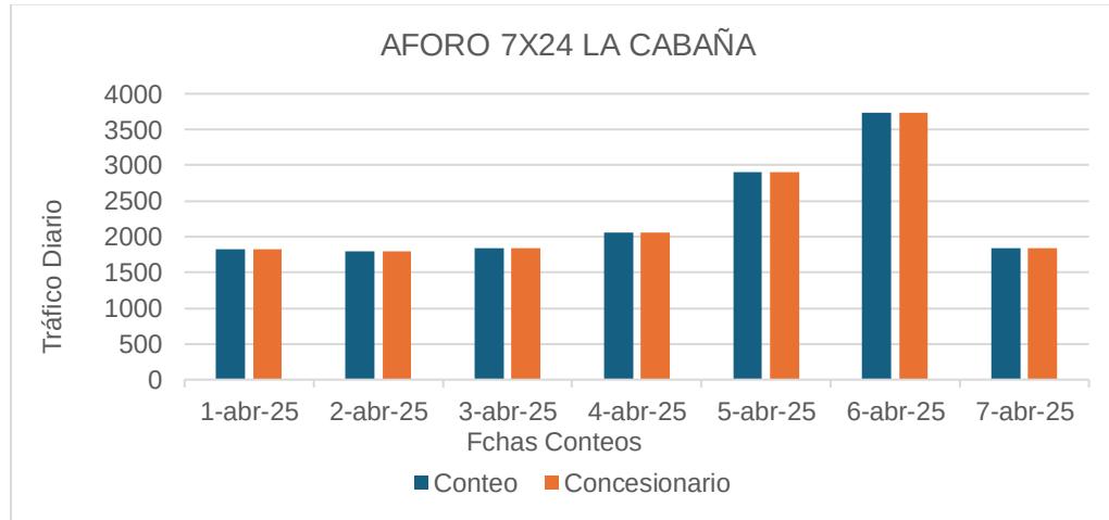
Figura 58 Comparativo Aforo 7x24 Peaje La Cabaña.
