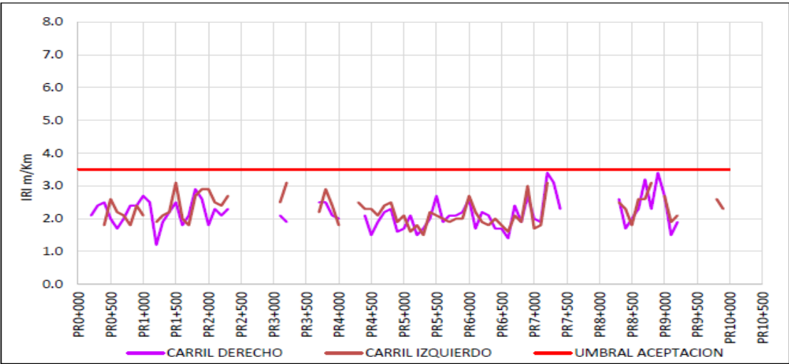
Figura 29 Evaluación E1 UF3A
