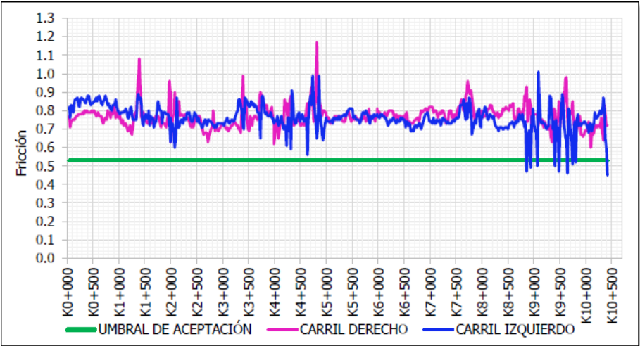
Figura 25 Evaluación E4 Fricción UF2A.
