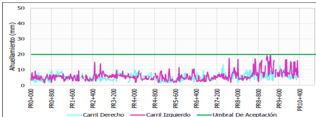
Figura 22 Evaluación E2 Ahuellamiento UF2A.
