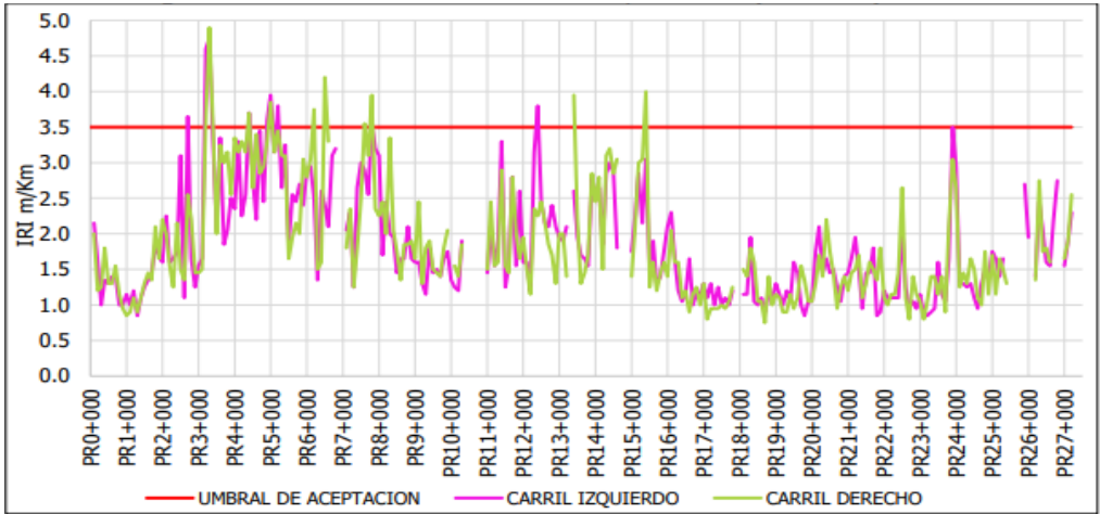
Figura 8 Evaluación E1 Iri UF1B.
