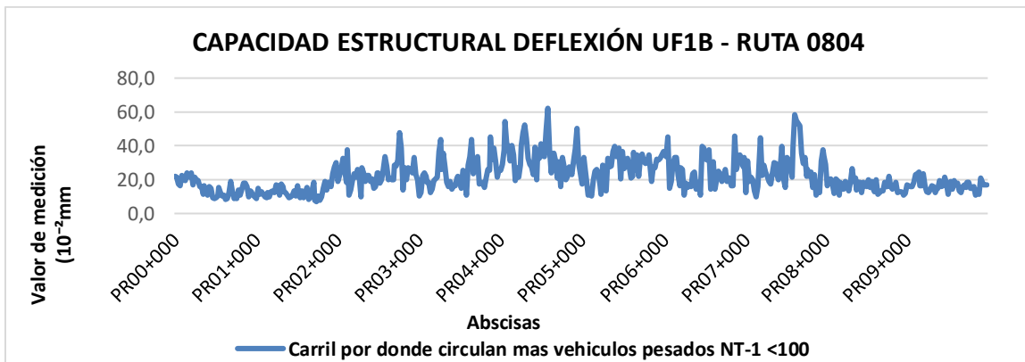
Figura 17 Evaluación E16 Capacidad Estructural UF1B
