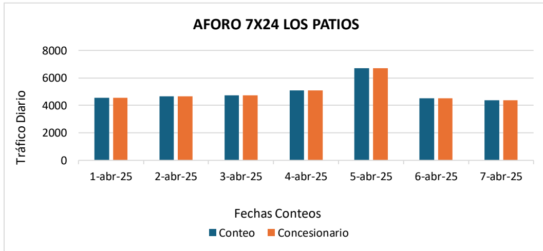
Figura 59 Comparativo Aforo 7x24 Peaje Los Patios
