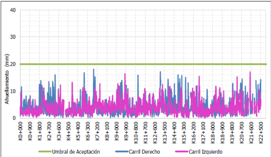
Figura 32 Evaluación E2 UF3B
