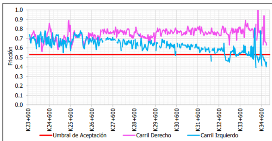
Figura 11 Evaluación E4 Fricción Transversal UF1A
