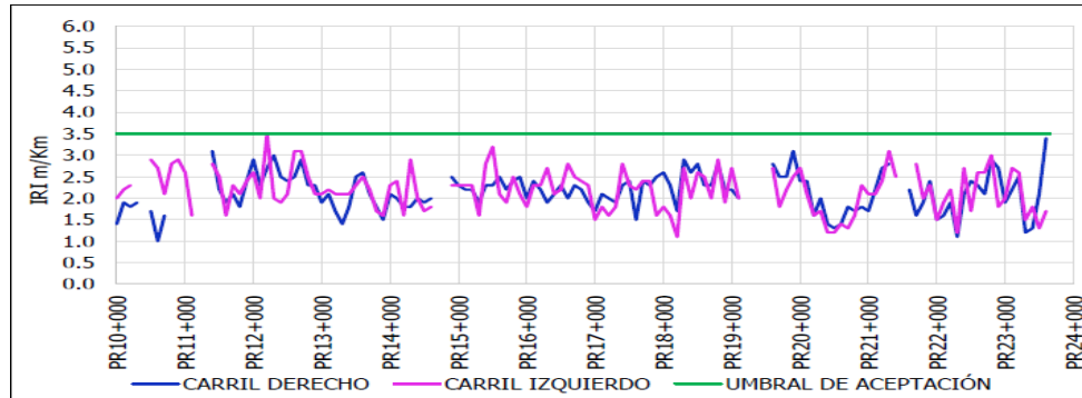
Figura 21 Evaluación E1 Iri UF2B.
