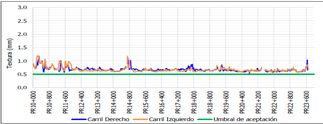
Figura 25 Evaluación E5 Textura UF2B
