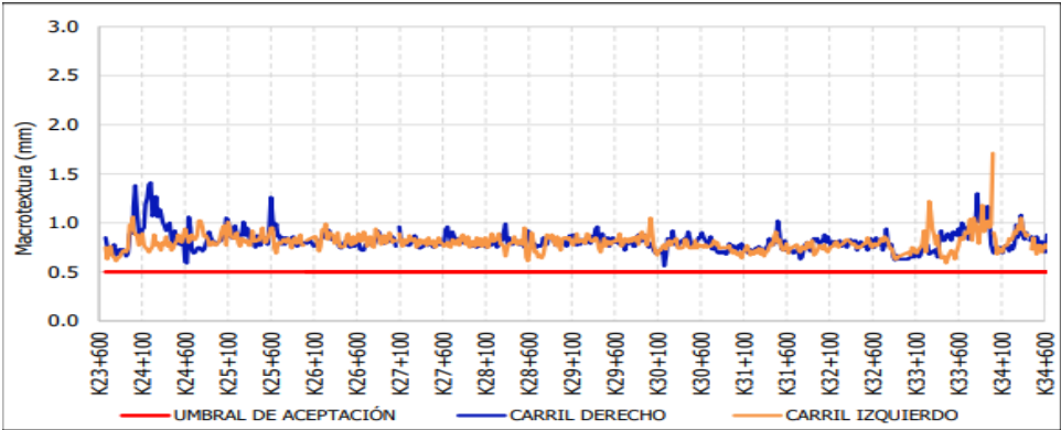
Figura 13 Evaluación E5 Textura UF1A
