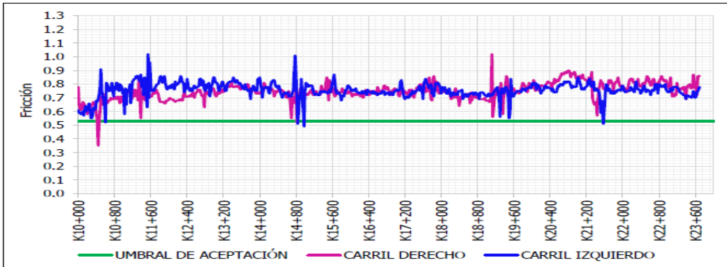
Figura 26 Evaluación E4 Fricción UF2B.
