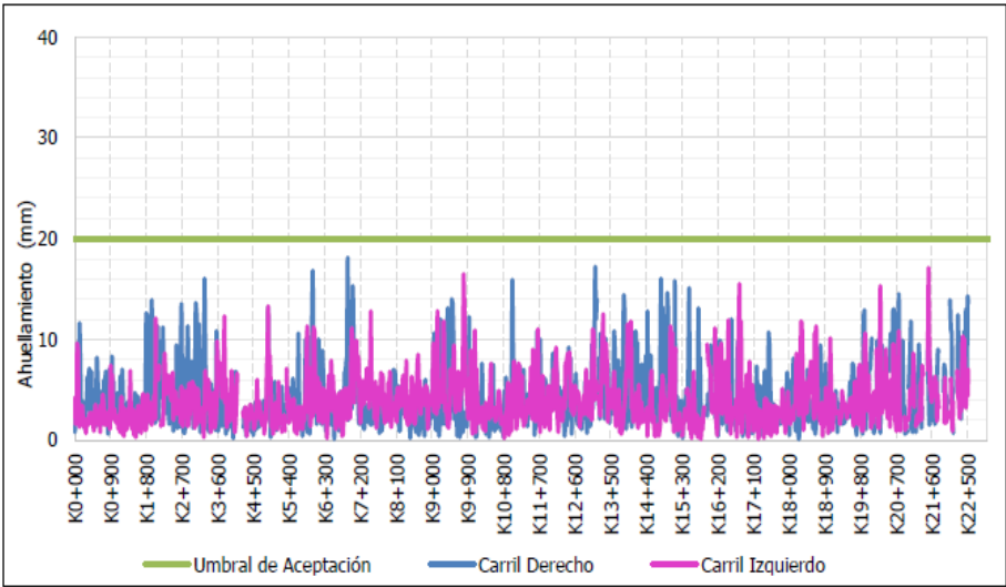
Figura 32 Evaluación E2 UF3B
