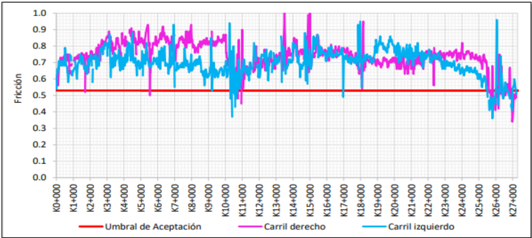
Figura 12 Evaluación E4 Fricción Transversal UF1B
