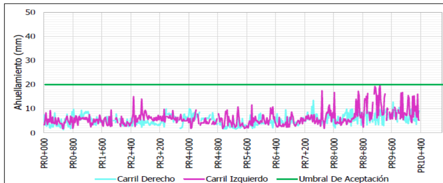
Figura 22 Evaluación E2 Ahuellamiento UF2A.
