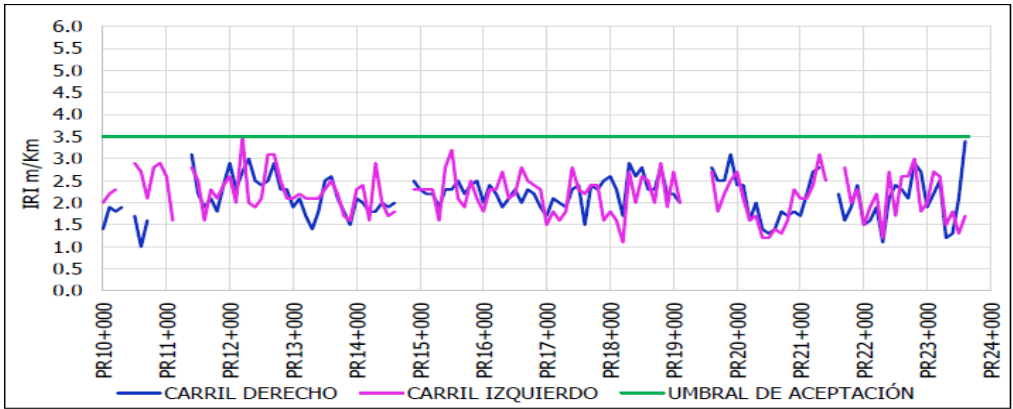
Figura 21 Evaluación E1 Iri UF2B.
