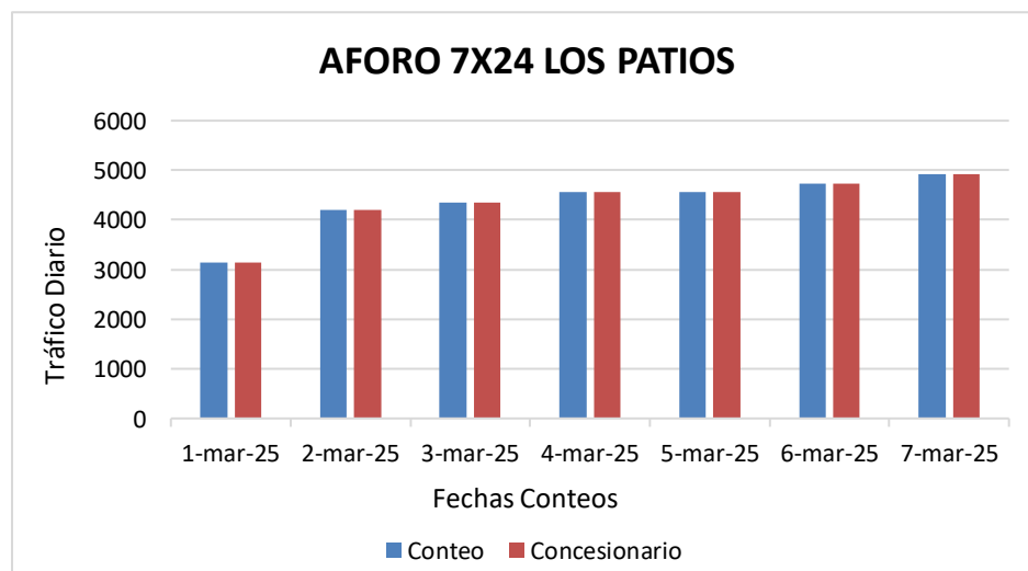
Figura 59 Comparativo Aforo 7x24 Peaje Los Patios
