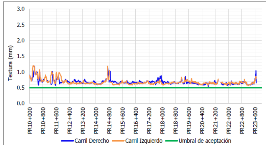
Figura 25 Evaluación E5 Textura UF2B
