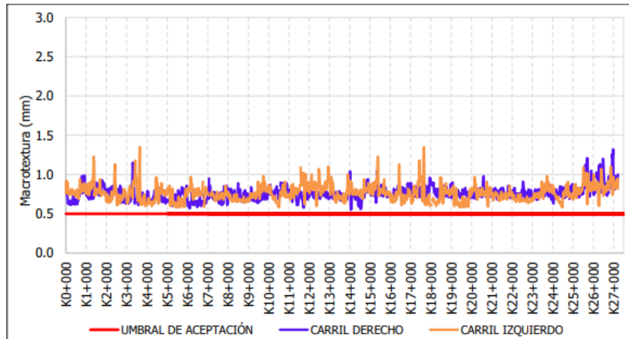
Figura 14 Evaluación E5 Textura UF1B
