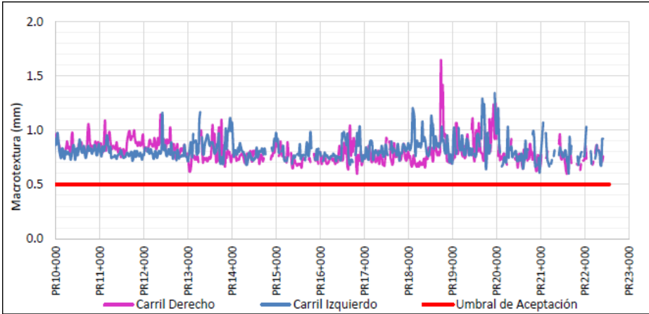
Figura 36 Comportamiento indicador E5 UF3A
