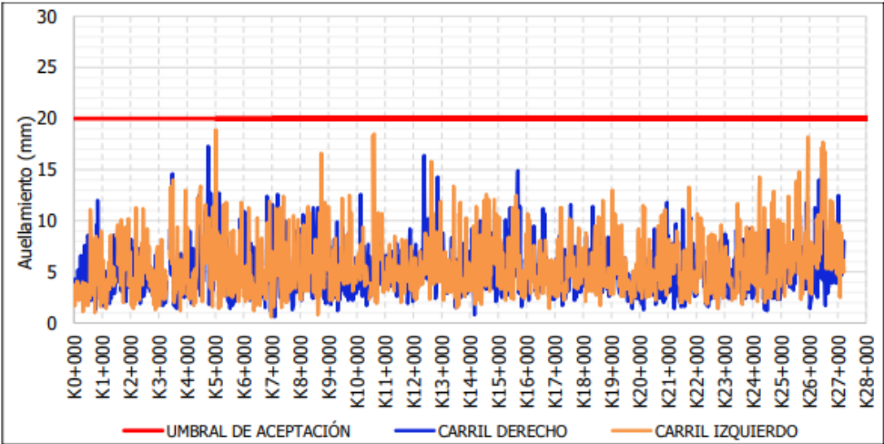
Figura 10 Evaluación E2 Ahuellamiento UF1B.
