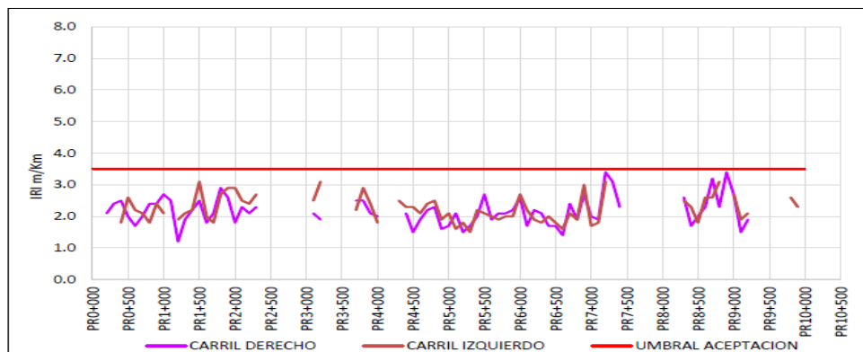
Figura 29 Evaluación E1 UF3A
