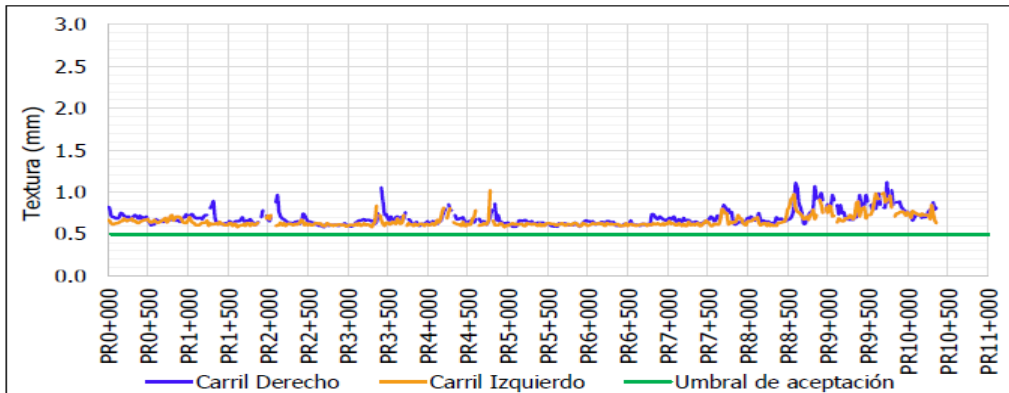
Figura 24 Evaluación E5 Textura UF2A
