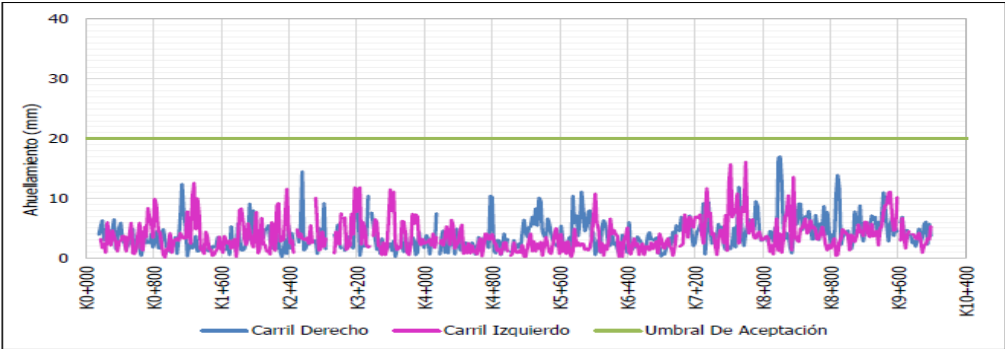
Figura 31 Evaluación E2 UF3A
