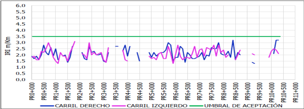
Figura 20 Evaluación E1 Iri UF2A
