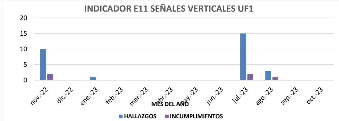
Figura 16 Comportamiento indicador E11 señalización vertical UF1.
