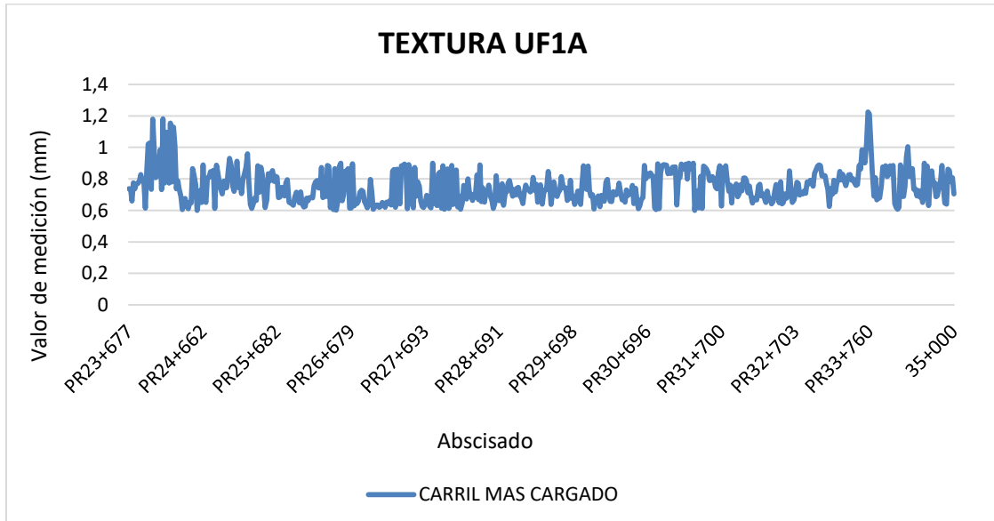
Figura 11 Comportamiento indicador E5 textura UF1A
