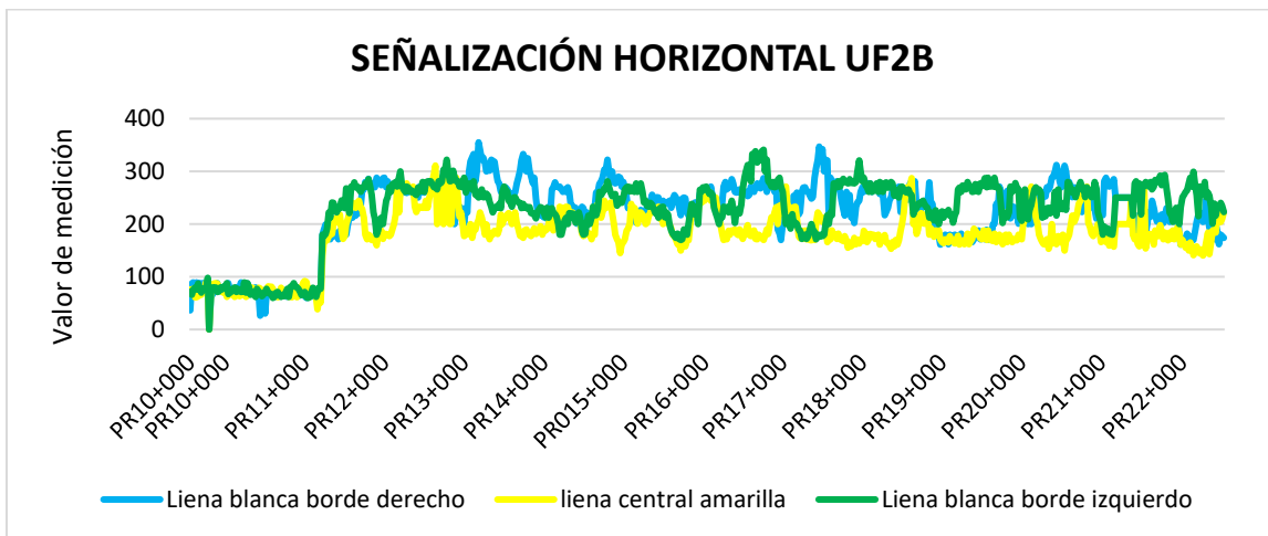
Figura 39 Comportamiento indicador E12 SEÑALIZACION HORIZONTAL
