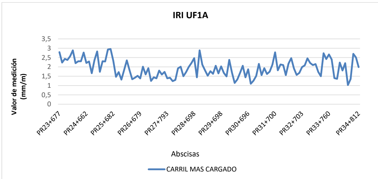
Figura 4 Comportamiento del indicador E1 IRI UF1A
