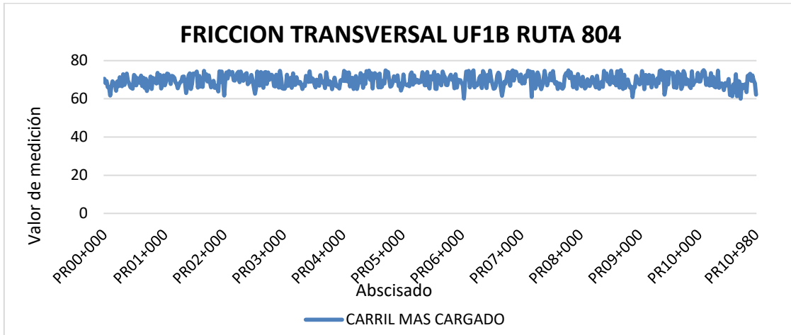
Figura 10 Comportamiento indicador E4 FRICCIÓN TRANSVERSAL UF1B
