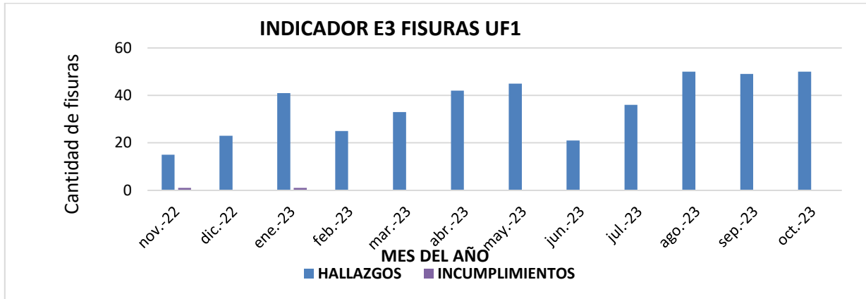
Figura 8 Comportamiento indicador E3 FISURAS UF1
