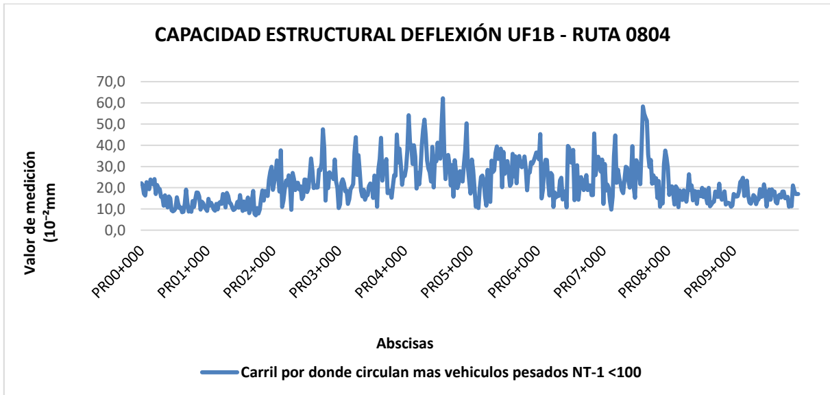
Figura 21 Comportamiento indicador E16 CAPACIDAD ESTRUCTURAL UF1B
