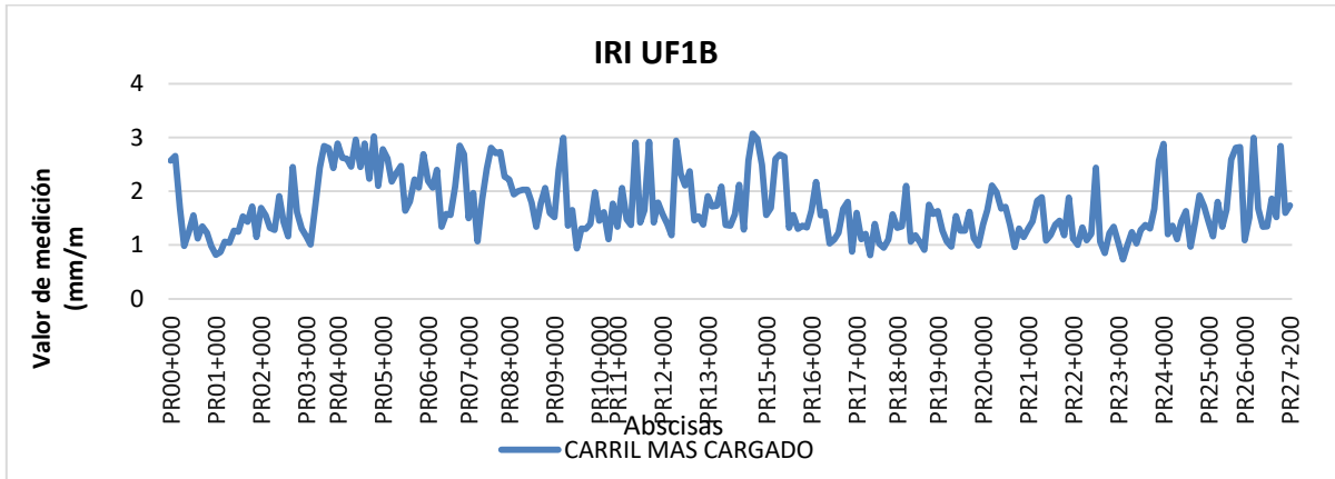
Figura 5 Comportamiento del indicador E1 IRI UF1B.
