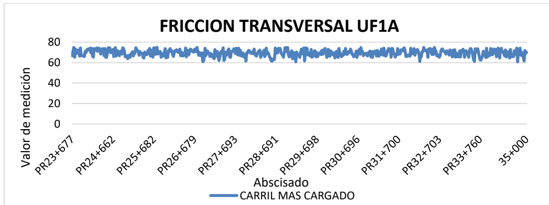
Figura 9 Comportamiento indicador E4 FRICCIÓN TRANSVERSAL UF1A
