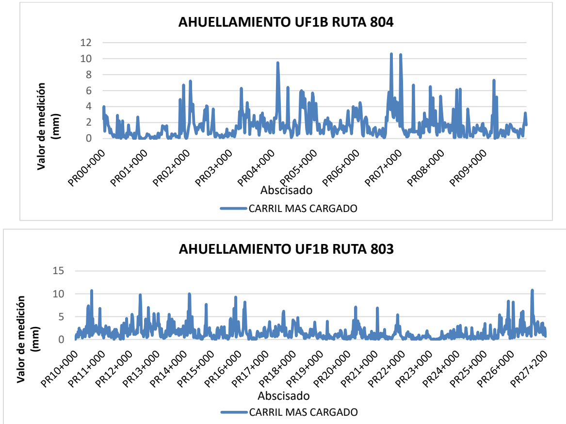
Figura 7 Comportamiento del indicador E2 AHUELLAMIENTO UF1B.
