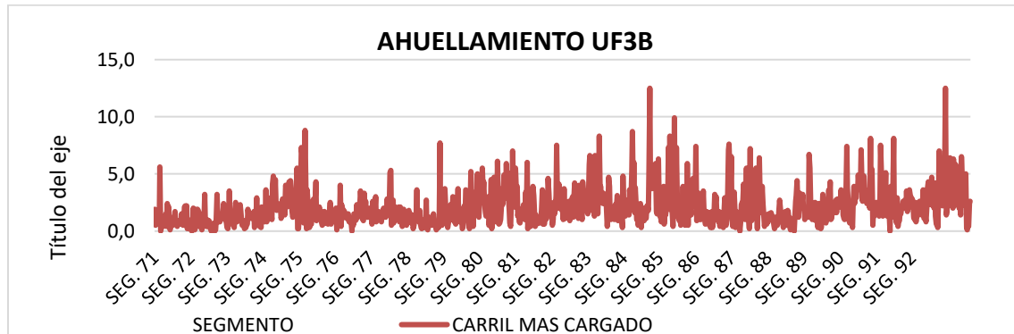
Figura 46 COMPORTAMIENTO INDICADOR E2 UF3B
