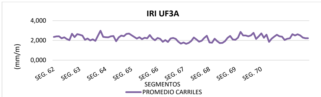
Figura 43 COMPORTAMIENTO INDICADOR E1 UF3A
