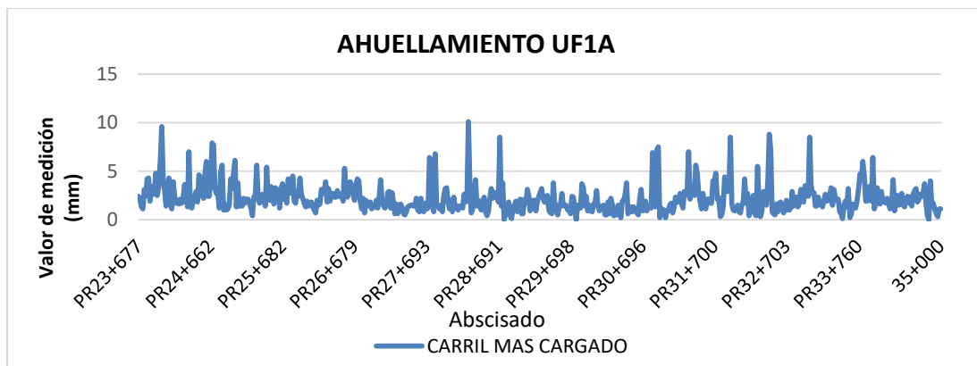
Figura 6 Comportamiento del indicador E2 AHUELLAMIENTO UF1A
