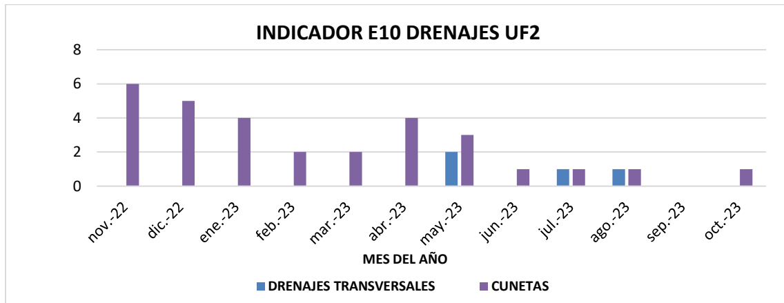
Figura 36 Comportamiento indicador E10 DRENAJES UF2.
