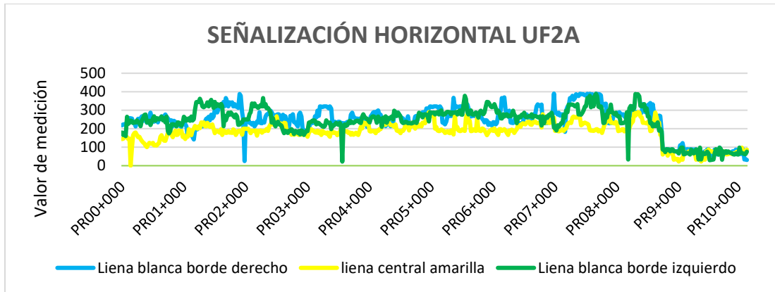
Figura 38 Comportamiento indicador E12 SEÑALIZACION HORIZONTAL
