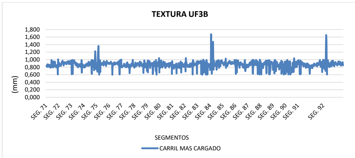
Figura 51 Comportamiento indicador E5 UF3B
