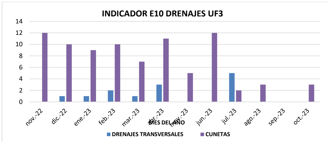
Figura 54 Comportamiento indicador E10 DRENAJES UF3.
