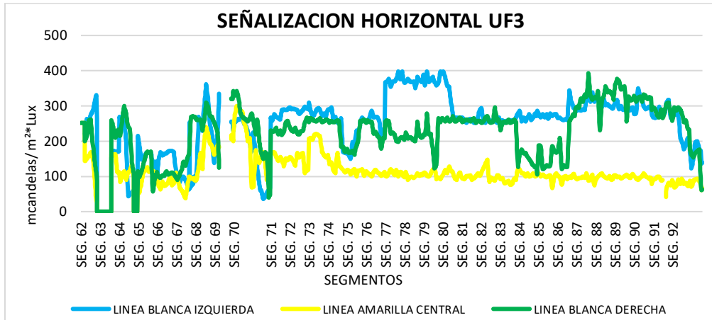
Figura 56 Comportamiento indicador E12 UF3
