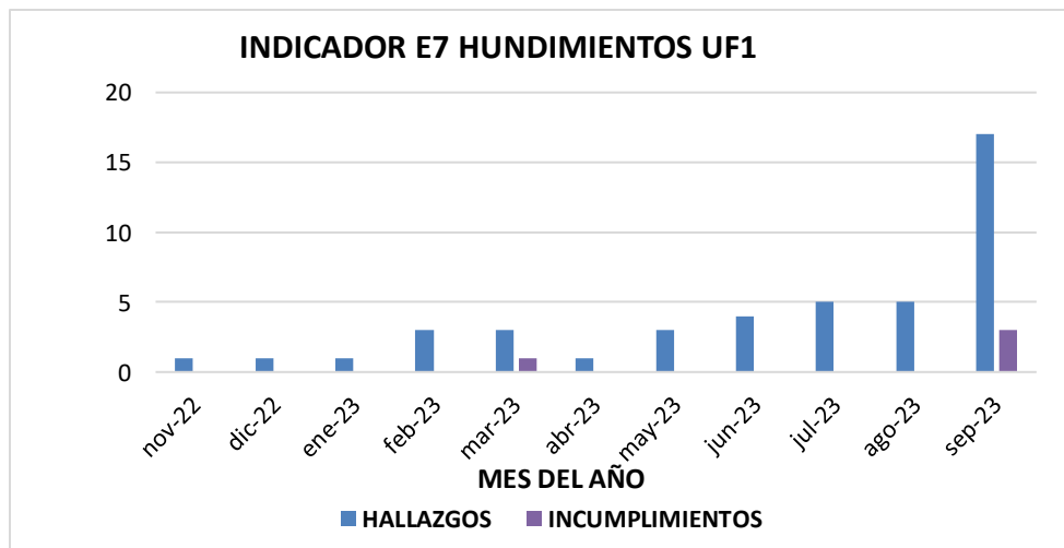
Figura 13 Comportamiento Indicador E7 HUNDIMIENTOS UF1
