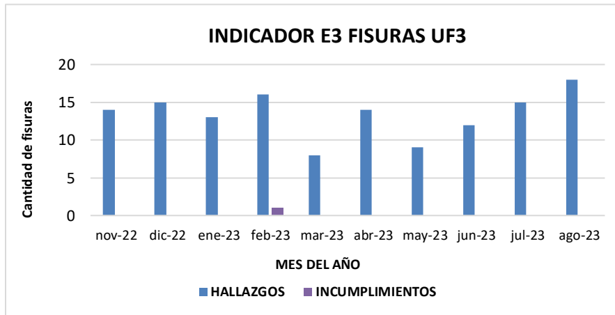
Figura 47 Comportamiento indicador E3 FISURAS UF3
