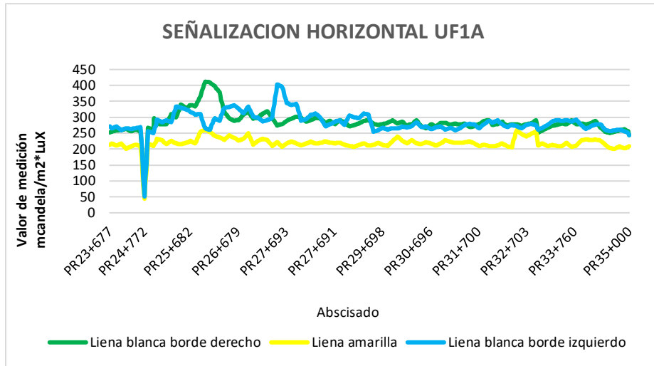
Figura 17 Comportamiento indicador E12 UF1A.
