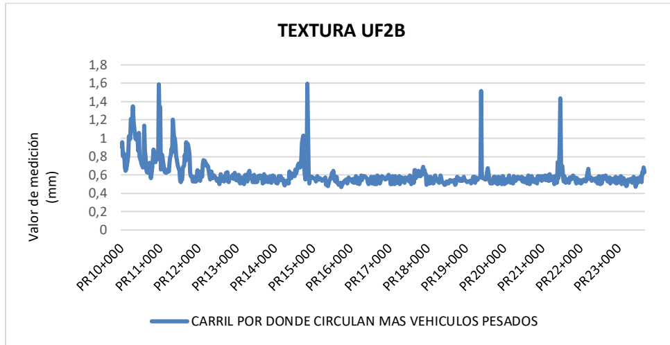
Figura 33 COMPORTAMIENTO INDICADOR E5 TEXTURA UF2B
