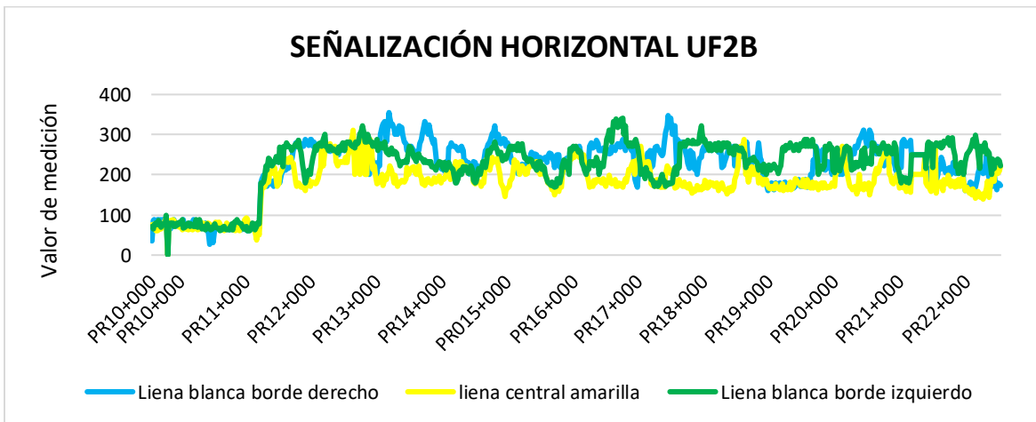
Figura 39 Comportamiento indicador E12 SEÑALIZACION HORIZONTAL
