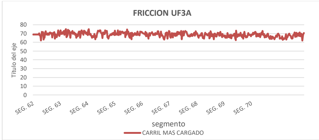
Figura 48 Comportamiento indicador E4 UF3A
