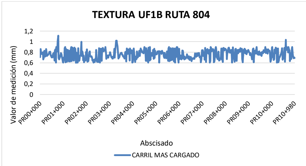
Figura 12 Comportamiento indicador E5 textura UF1B
