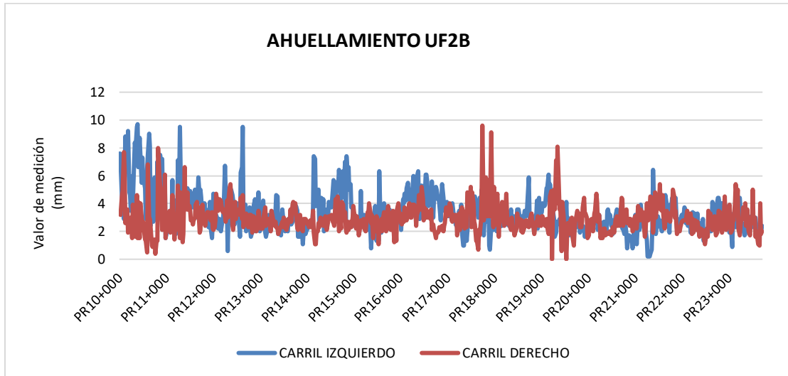
Figura 28 COMPORTAMIENTO INDICADOR E2 AHUELLAMIENTO UF2B.
