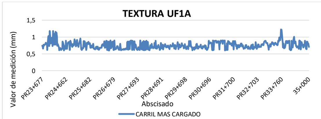
Figura 11 Comportamiento indicador E5 textura UF1A
