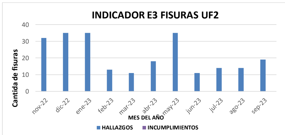
Figura 29 Comportamiento indicador E3 FISURAS UF2.
