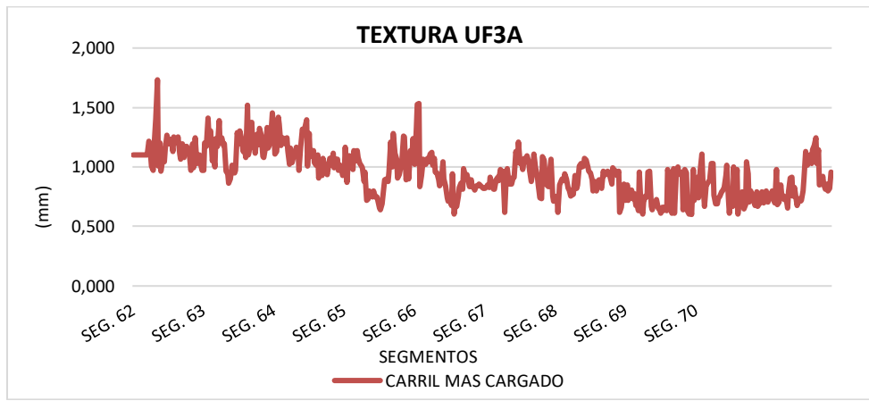
Figura 50 Comportamiento indicador E5 UF3A
