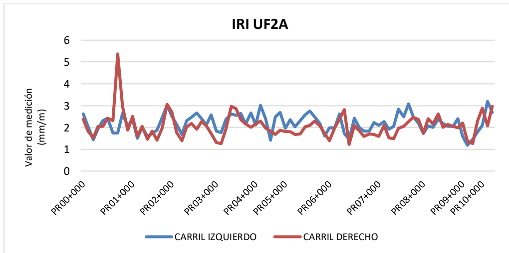
Figura 25 COMPORTAMIENTO INDICADOR E1 IRI UF2A
