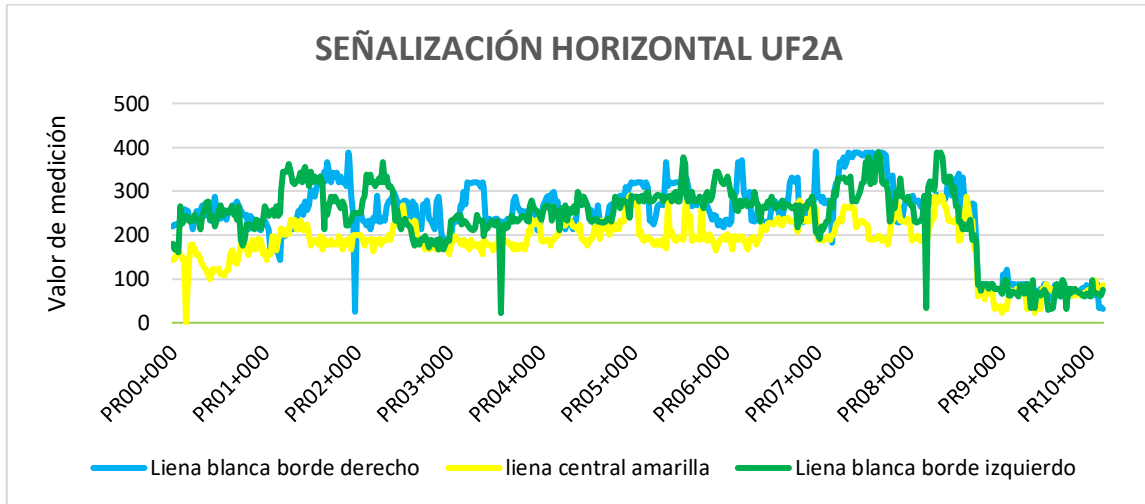
Figura 38 Comportamiento indicador E12 SEÑALIZACION HORIZONTAL
