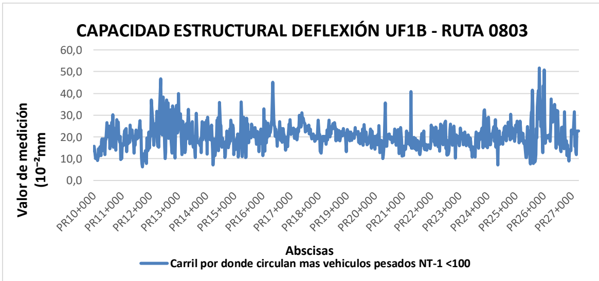
Figura 22 Comportamiento indicador E16 CAPACIDAD ESTRUCTURAL UF1B
