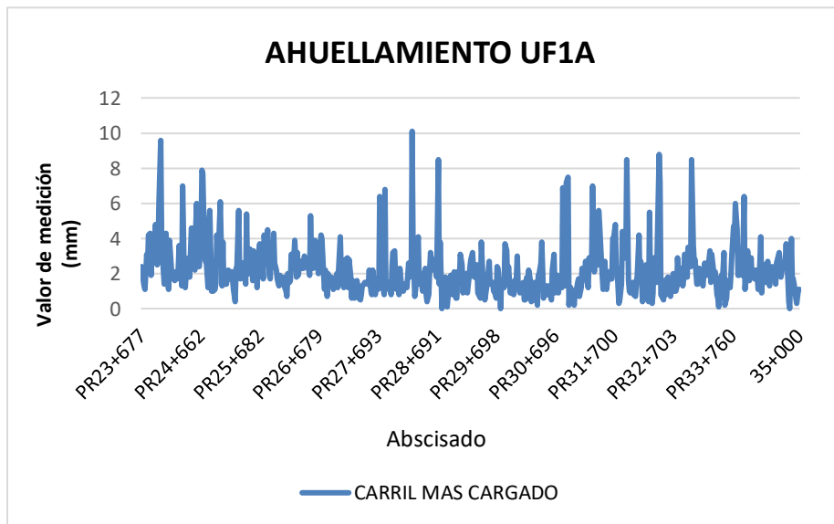
Figura 6 Comportamiento del indicador E2 AHUELLAMIENTO UF1A
