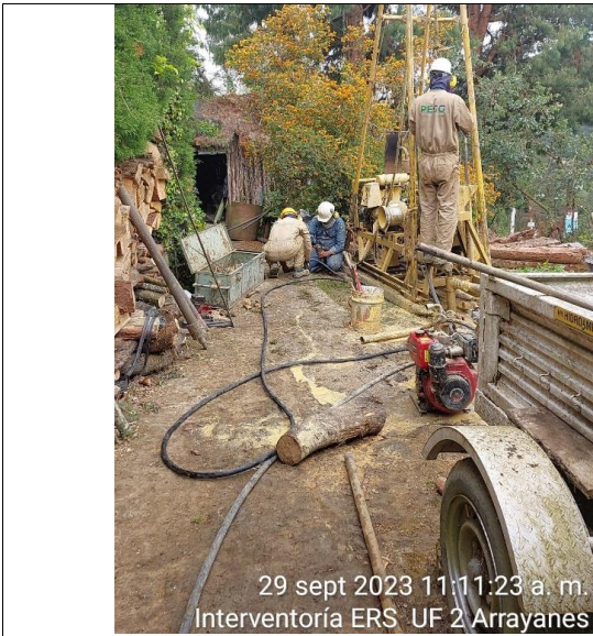
Ilustración 15 Máquina perforadora en el punto 3 y trabajos de campo.
