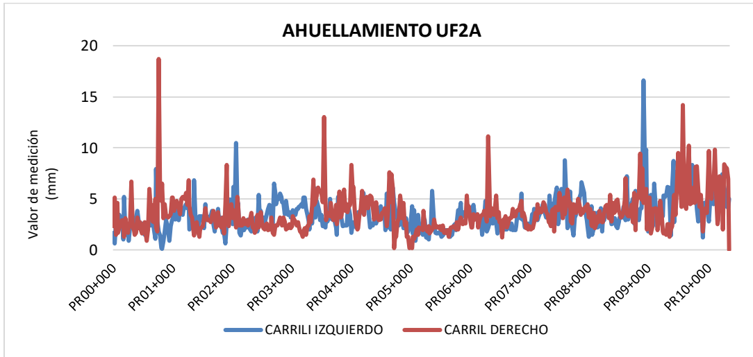
Figura 27 COMPORTAMIENTO INDICADOR E2 AHUELLAMIENTO UF2A.
