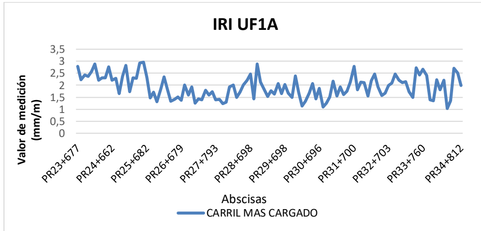
Figura 4 Comportamiento del indicador E1 IRI UF1A
