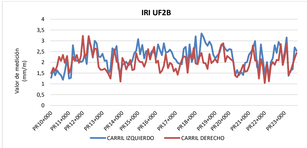
Figura 26 COMPORTAMIENTO INDICADOR E1 IRI UF2B.
