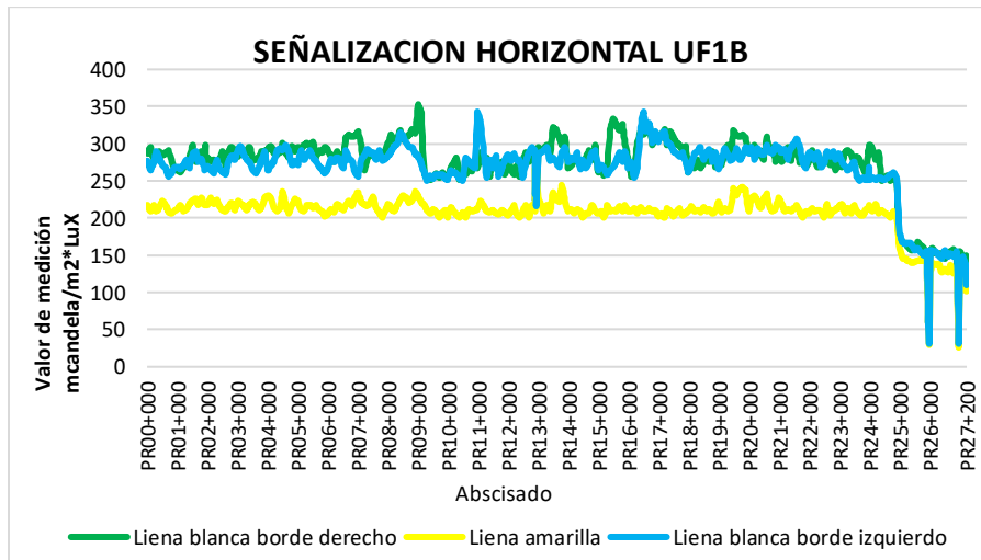
Figura 18 Comportamiento indicador E12 UF1B
