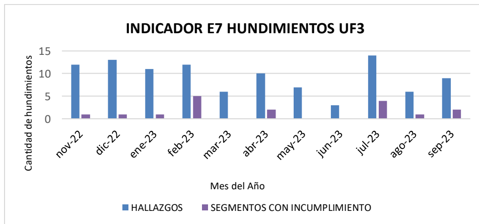
Figura 52 Comportamiento indicador E7 HUNDIMIENTOS UF3.
