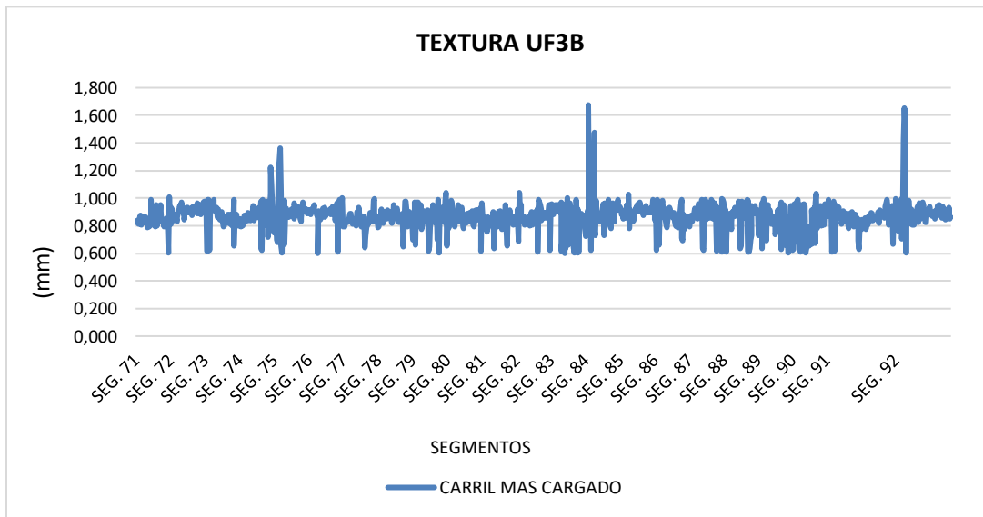
Figura 51 Comportamiento indicador E5 UF3B
