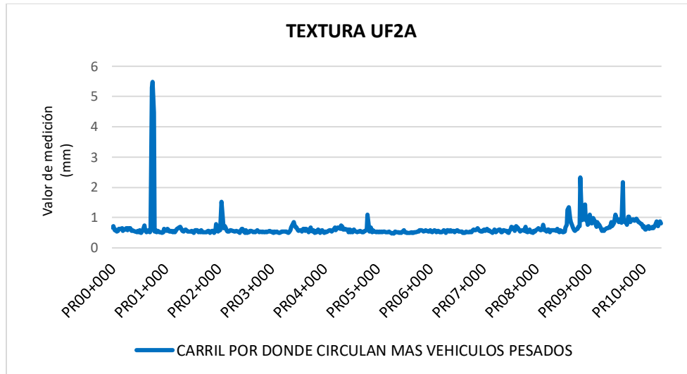
Figura 32 COMPORTAMIENTO INDICADOR E5 TEXTURA UF2A
