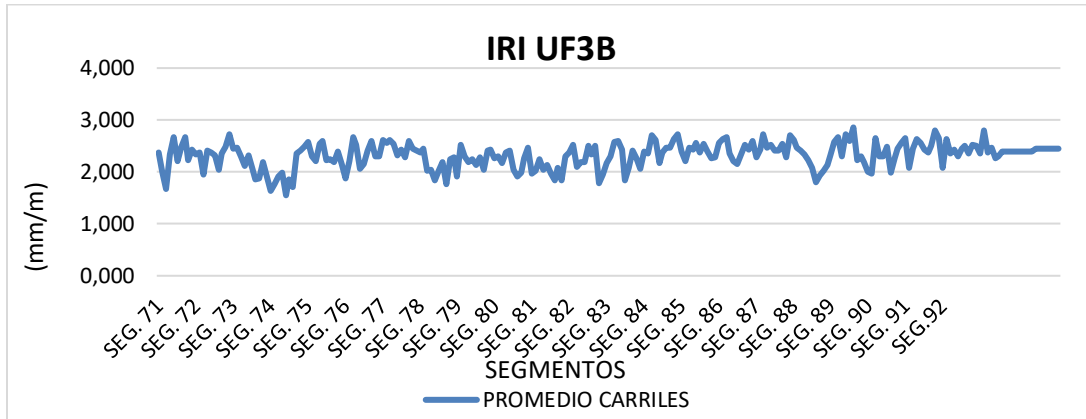
Figura 44 COMPORTAMIENTO INDICADOR E1 UF3B
