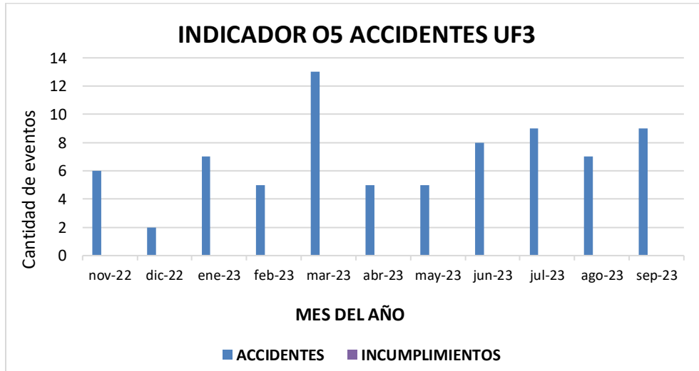
Figura 59 COMPORTAMIENTO INDICADOR 05 UF3.
