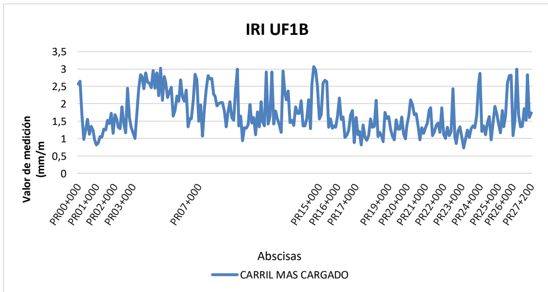
Figura 5 Comportamiento del indicador E1 IRI UF1B.
