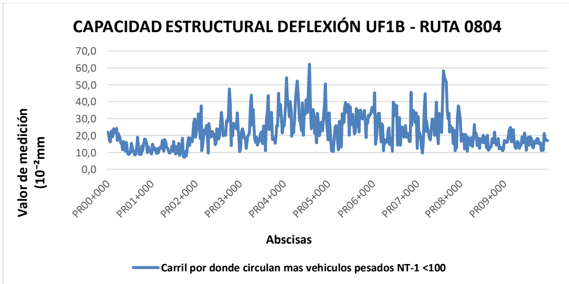
Figura 21 Comportamiento indicador E16 CAPACIDAD ESTRUCTURAL UF1B
