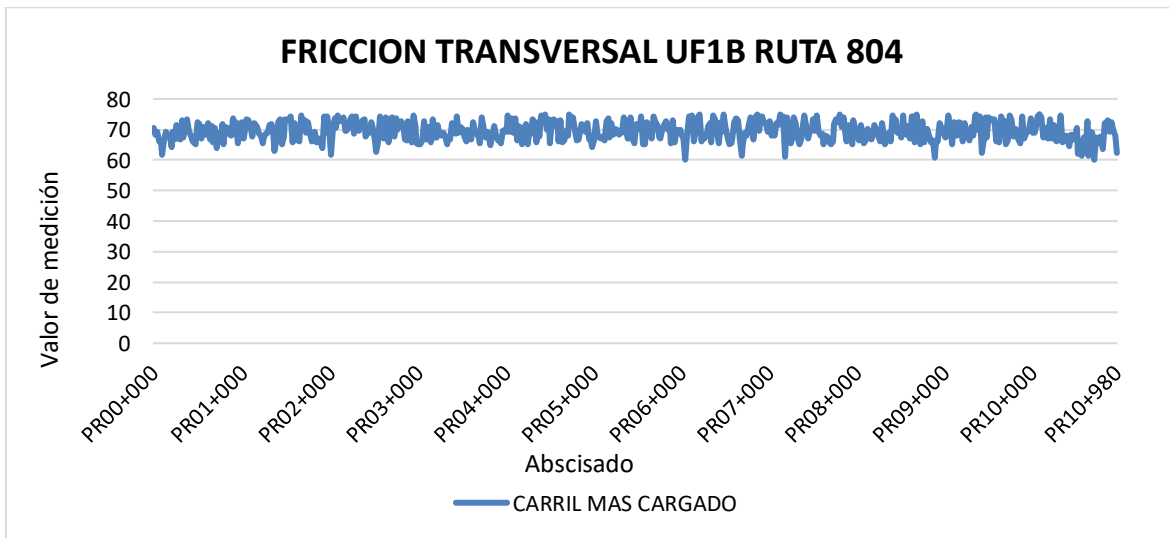
Figura 10 Comportamiento indicador E4 FRICCIÓN TRANSVERSAL UF1B
