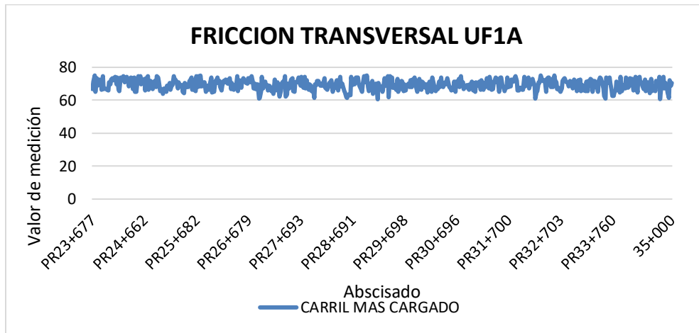
Figura 9 Comportamiento indicador E4 FRICCIÓN TRANSVERSAL UF1A
