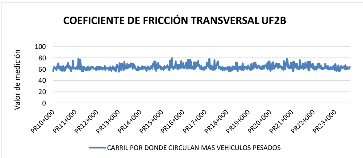
Figura 31 COMPORTAMIENTO INDICADOR E4 FRICCIÓN UF2B
