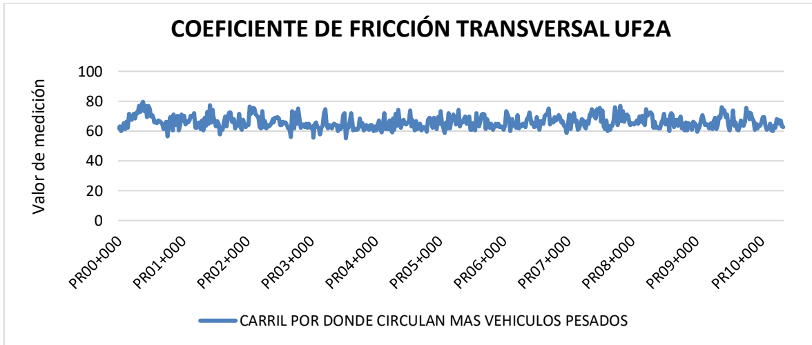
Figura 30 COMPORTAMIENTO INDICADOR E4 FRICCIÓN UF2A
