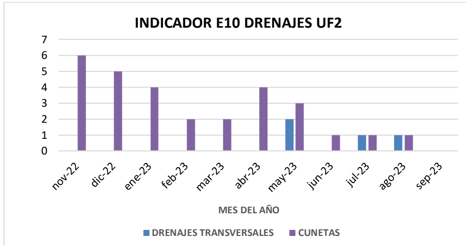
Figura 36 Comportamiento indicador E10 DRENAJES UF2.
